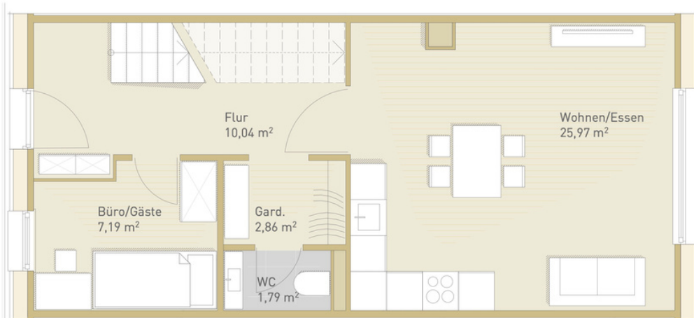
große Wohnung
