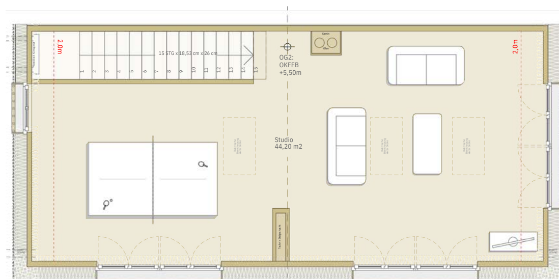
2. Obergeschoss
